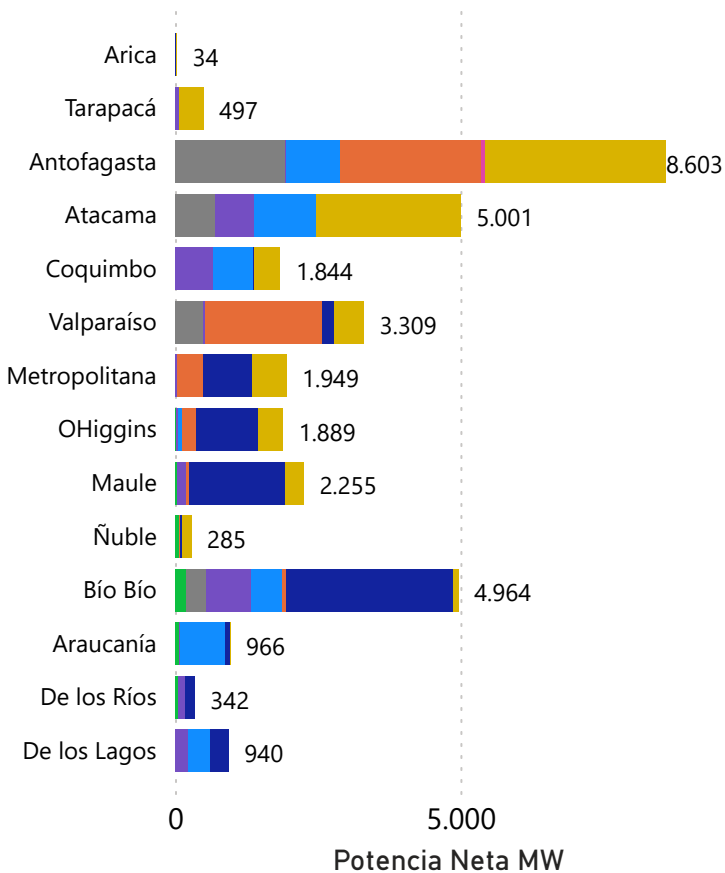
Capacidad instalada total a 2023
